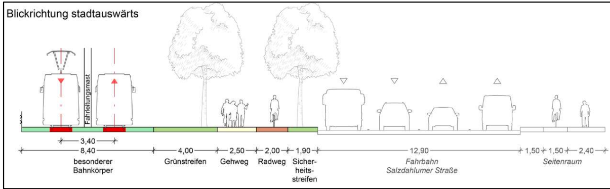
Abbildung 6-21: Projektteil Heidberg/Salzdahlumer Straße, Querschnitt Salzdhahler Straße, Stand Machbarkeitsuntersuchung
