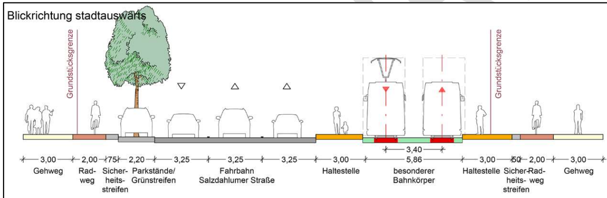
Abbildung 6-22: Projektteil Heidberg/Salzdahlumer Straße, Querschnitt Salzdhahler Straße - Haltestelle im Bereich Bebelhof, Stand Machbarkeitsuntersuchung
